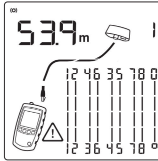
c) Kablo 3 ve 4 karışmış
