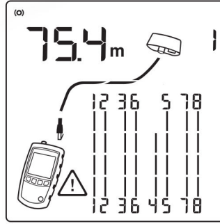
a) Kablo 4 blendajında açık devre
