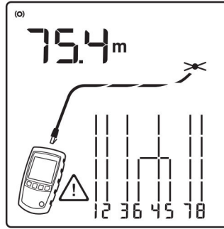
b) Kablo 6 ve 5 kısa devre
