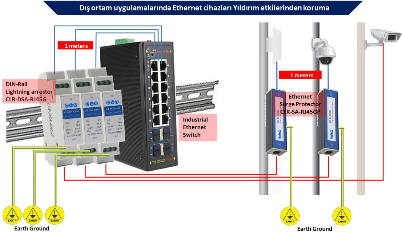
Resim 1 Dış ortam uygulamalarında ethernet cihazları yıldırım etkilerinden koruma - Lightning Protection
